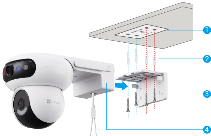
圖 1 天花板安裝
